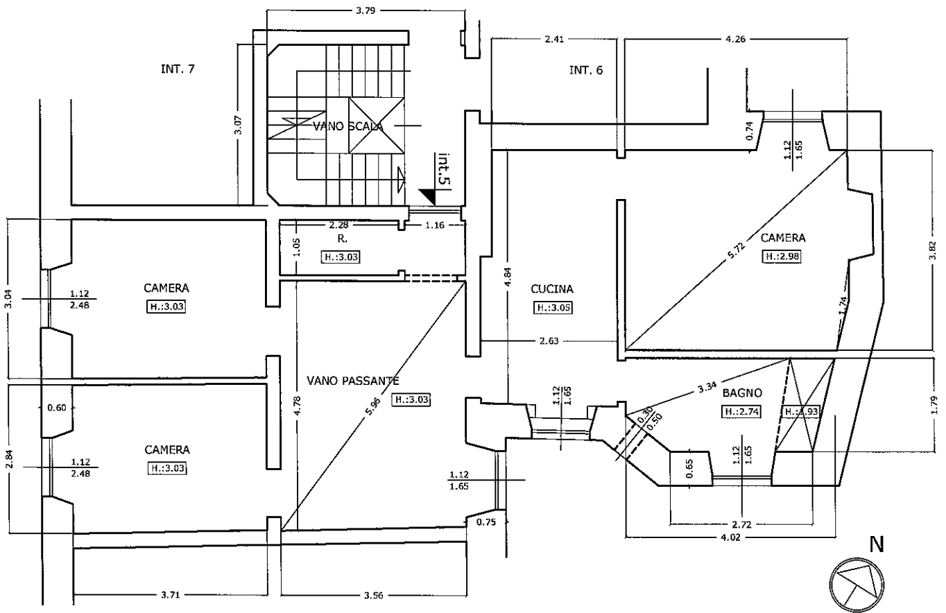
Planimetria quotata Scala 1:100
