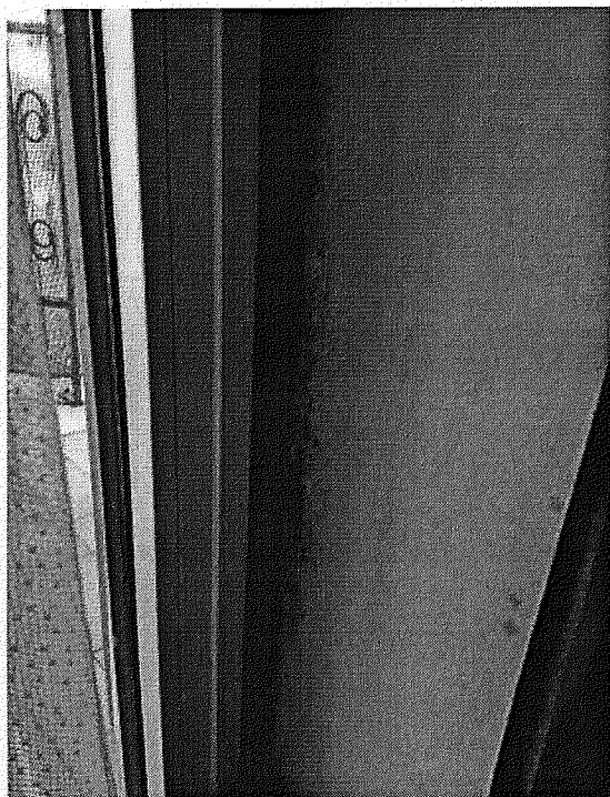
Foto 11-12: macchie e distacchi dovuti a condensa e infiltrazioni
