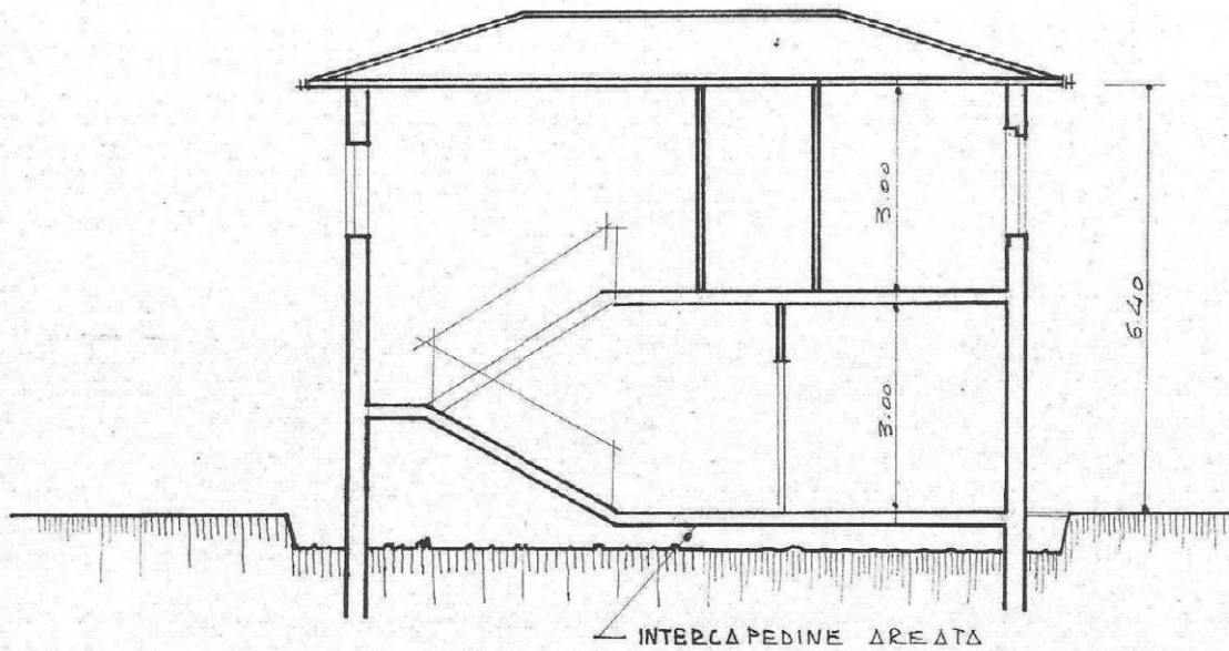
SEZIONE Δ-Δ
