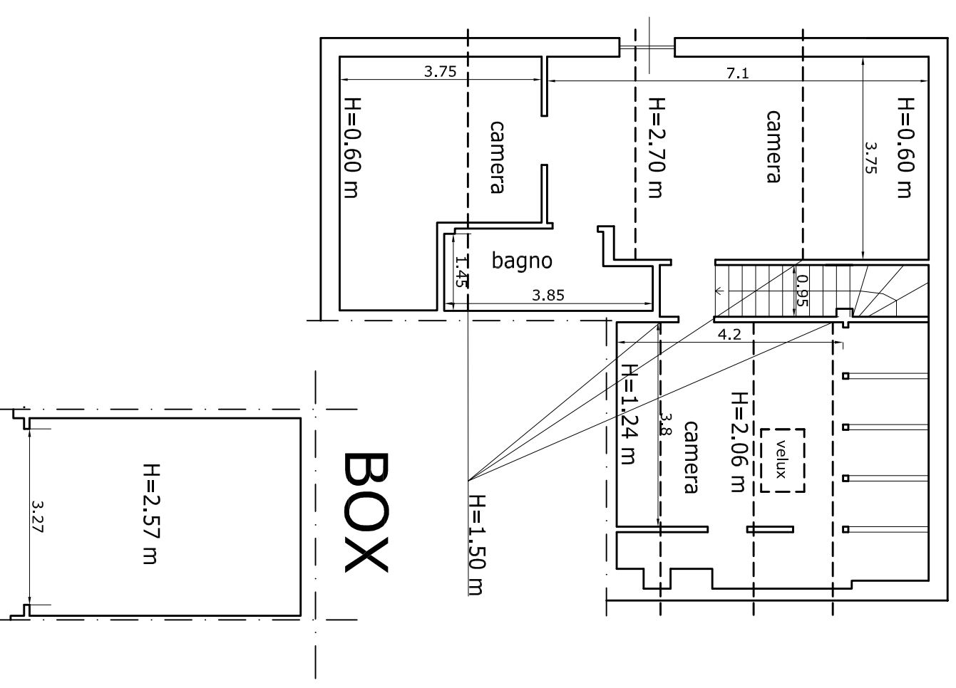
PIANO SOTTOTETTO
